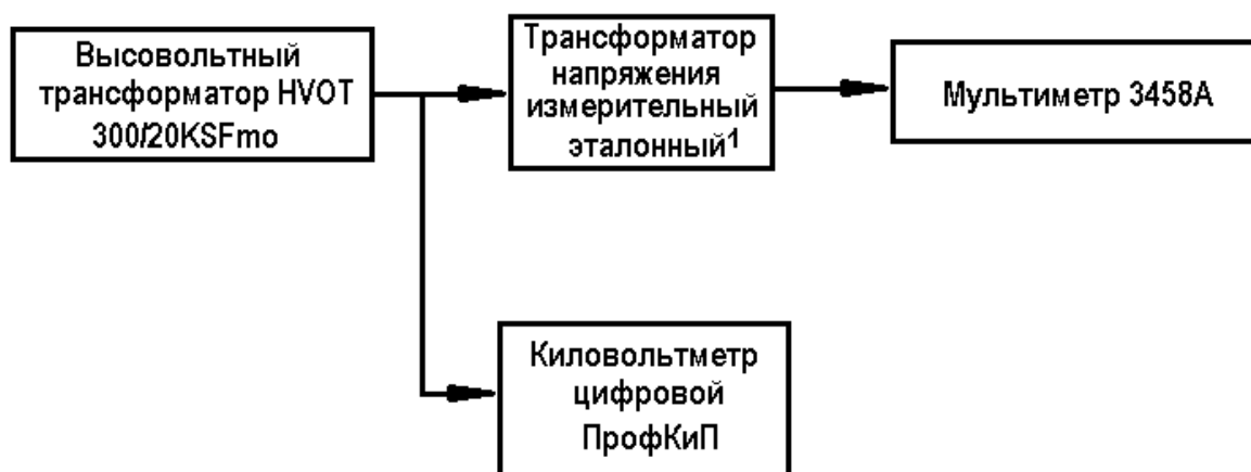
Рисунок 1-Структурная схема подключения приборов для определения относительной погрешности измерения среднеквадратических значений напряжения переменного тока синусоидальной формы частотой 50 Гц.
